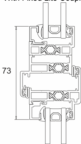
Coupling Bar
